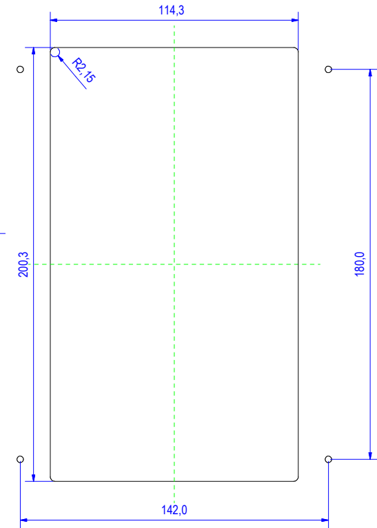
Ausschnitt und Bolzenbild Schweißbolzen M3x16mm
