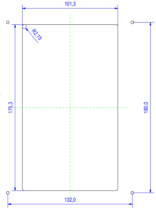
Ausschnitt und Bolzenbild Schweißbolzen M3x16mm
